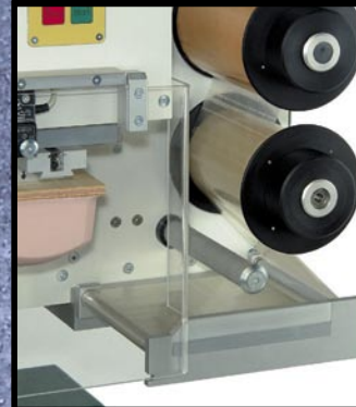
Automatische Tamponreinigung
